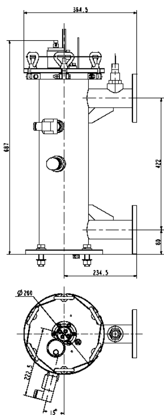
UV 灭菌反应器外形尺寸图
